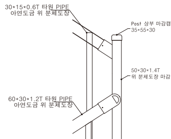
A - 횡주관 고정 상세도
