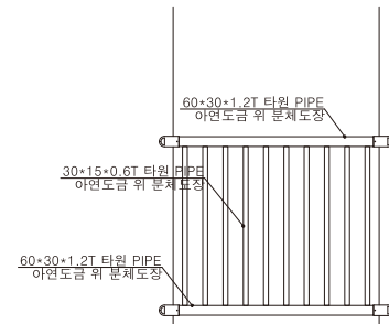
창보호난간 입면도
