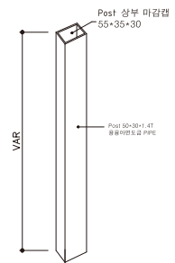
D - Post 상세도
