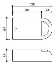
B' - 연결부속 상세도
