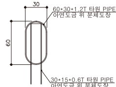
C - 횡주관 단면상세도
